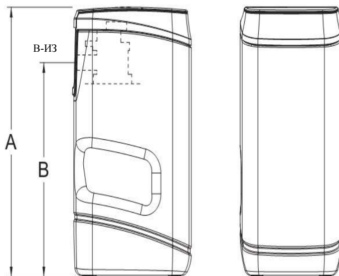
ВИД СБОКУ
